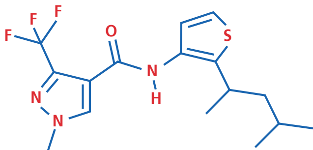
Συντακτικός τύπος του penthiopyrad
