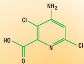
aminopyralid
