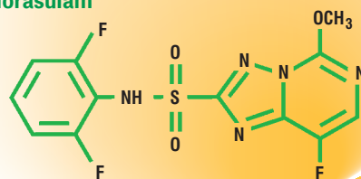
florasulam
